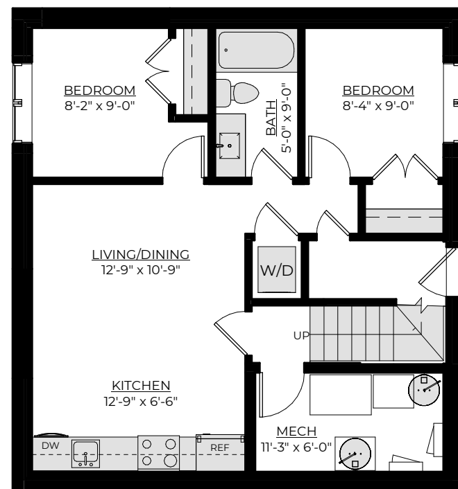
Optional Basement Suite 619 ft 2
